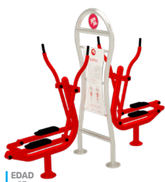
EDAD +13 Ejercitador Elíptica Forte EJE-FO-08-00 Largo: 2.95 m Ancho: 0.90 m Alto: 2.00 m Área mínima: 4.00 m x 1.90 m Usuarios: 2 personas
