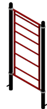
Ejercitador Pared Sueca y 2 Postes EJE-ID-23-00 Largo: 1.20 m Ancho: 0.40 m Alto: 2.60 m Área mínima: 2.20 m x 1.40 m Usuarios: 1 persona
