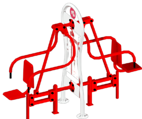
EDAD +13 Ejercitador Pecho Forte EJE-FO-11-00 Largo: 2.55 m Ancho: 0.70 m Alto: 2.00 m Área mínima: 3.60 m x 1.90 m Usuarios: 2 personas
