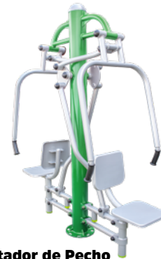
EDAD +13 Ejercitador Barras Paralelas OK Doble OKST-S03X Largo: 1.85 m Ancho: 0.55 m Alto: 1.60 m Área mínima: 2.45 m x 1.60 m Usuarios: 2 personas
