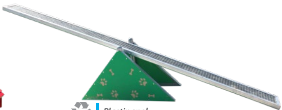
Balancín Canino CAN-PL-10-00 Dimensiones: L: 3.60 m An: 0.50 m Al: 1.10 m Área mínima: 4.60 m x 1.50 m Material: Acero y plastipanel
