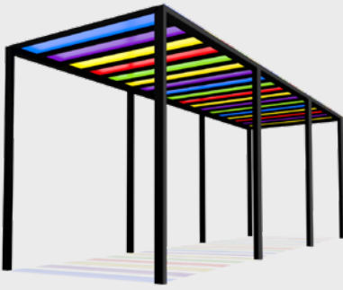
Techo Sombra de Color 12 Acrílico TEC-AC-01-00 Descripción: Techo de Acero con acrílico de colores. Medidas: 7.30 m x 1.60 m x 2.65 m Materiales: Acero y acrílicos de colores.
