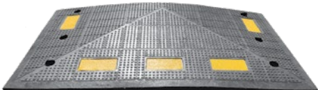
Tardo Cabecero Hembra LEPDM-HEM Dimensiones: L: 0.50 m An: 0.90 m Al: 0.6 m Peso: 16.5 Kg Material: Hule
