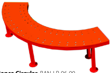
Banca Circular BAN-LP-06-00 Dimensiones: L: 1.80 m An: 0.70 m Al: 0.45 m Ancho asiento: 0.35 m Capacidad: 3 Personas Material: Lámina troquelada *Sistema modular
