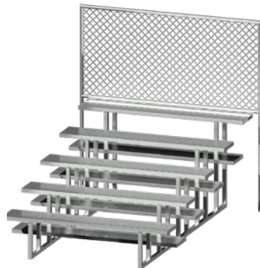
Gradas 5 Asientos y 4 Descansa Pies DEP-MO-04-00 Largo: 2.75 m Ancho: 1.90 m Alto: 2.10 m Área mínima: 3.05 m x 2.90 m Usuarios: 24 personas
