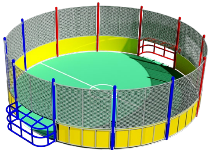
Cancha Circular de Fútbol Rápido DEP-00-12-00 Largo: 8,05 m Ancho: 7,05 m Alto: 2,25 m Usuarios: 6 niños Incluye pasto
