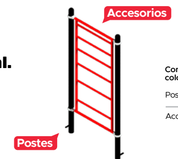
EDAD +13 Ejercitador Pasamanos y 6 Postes EJE-EST-02-00 Largo: 6,35 m Ancho: 1,20 m Alto: 2,60 m Área mínima: 7,35 m x 2,30 m
