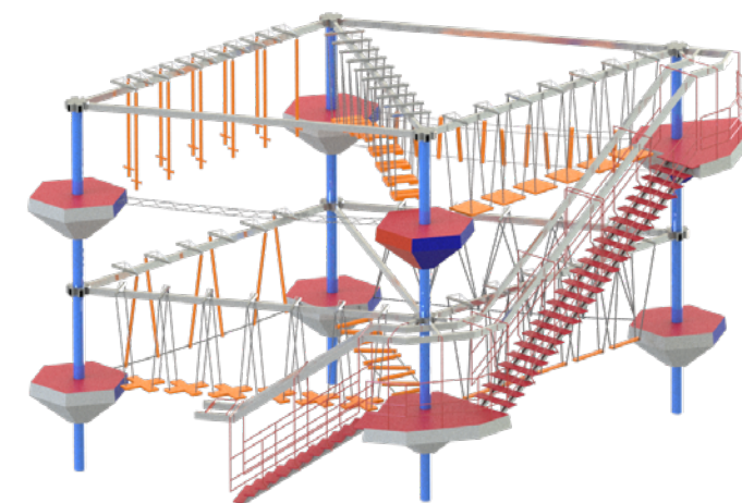
ROPES COURSE AX 4.10 | HX-AX4-10 Largo: 14 m Ancho: 9 m Alto: 6 m Área segura: 17.5 m x 11.5 m Las medidas no incluyen la escalera de acceso.
