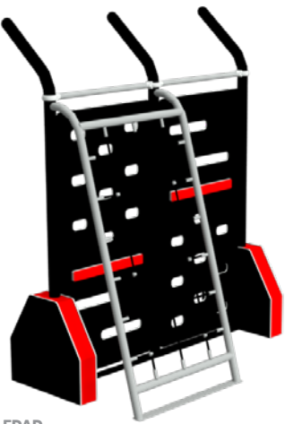
EDAD +13 Pared Militar EJE-ID-52-00 Largo: 2.40 m Ancho: 1.45 m Alto: 2.85 m Área mínima: 6.00 m x 1.75 m Usuarios: 2 personas
