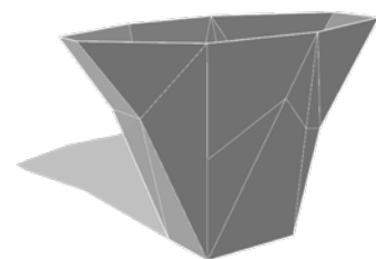
BOULDER 360° GIBRALTAR | HXC-BG MEDIUM: 14 m² escalables. Ancho: 1.25 m, Largo: 3.75 m, Alto: 2.50 m. LARGE: 28 m² escalables. Ancho: 2.50 m, Largo: 5 m, Alto: 3.25 m.
