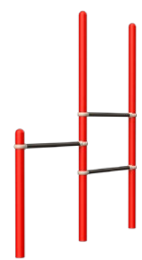
EDAD +13 Ejercitador Barras de Estiramiento EJE-EST-10-00 Largo: 2,30 m Ancho: 0,10 m Alto: 2,20 m Área mínima: 3,30 m x 1,40 m
